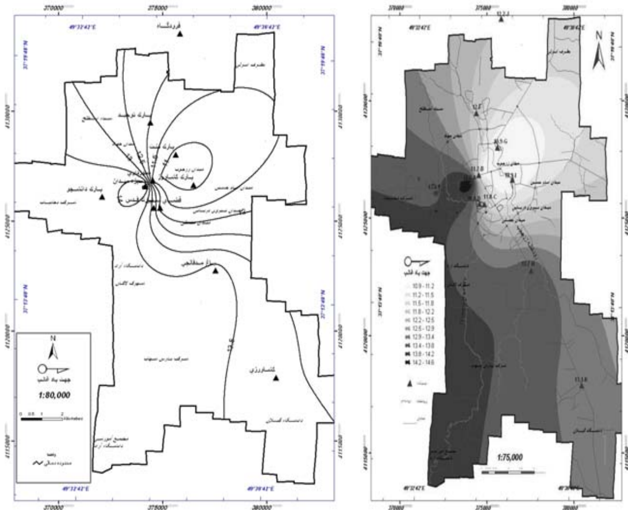
شکل شماره ۴- نقشه همدمای میانگین حداکثر دمای اسفند ماه ۱۳۸۵ شهر رشت
